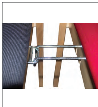
Reihenverbindung, als Metallbügel ausziehbar, verchromt RVA-CH 27,37 23,-*
